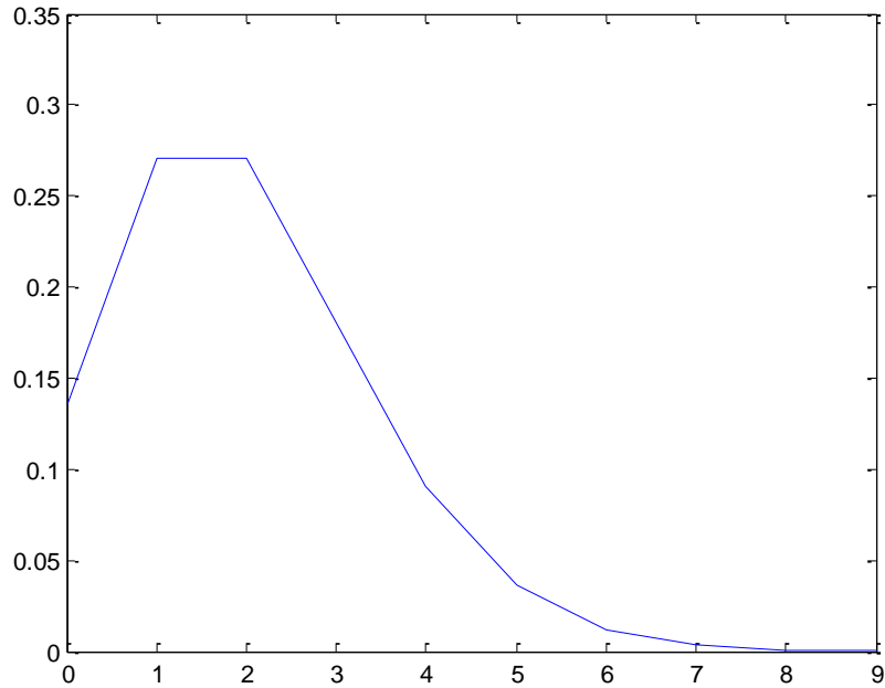
شكل رقم (7): دالة احتمال بواسون لقيم x عند \mu=2
