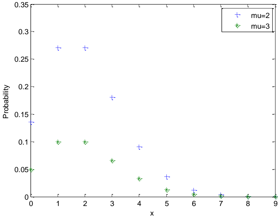
شكل رقم (8): مقارنة الشكلين عند \mu=2 , \mu=3 .
