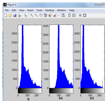
شكل رقم (7): تغير مركز التوزيع بعد الاضافة و الطرح
